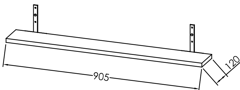
POLICA OG 90 WH
